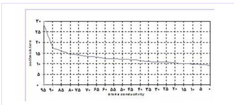
شکل ۱: منحنی کالیبراسیون
