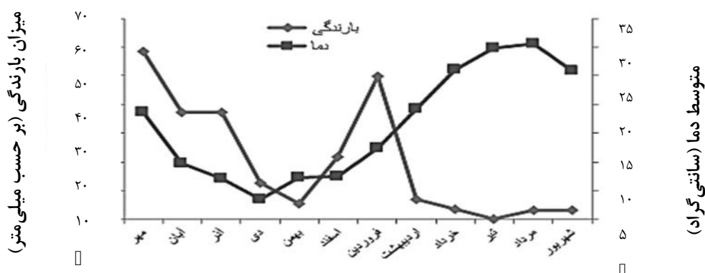
شکل ۱: نمودار آمبروترمیک محل آزمایش در سال زراعی ۹۴-۱۳۹۳
