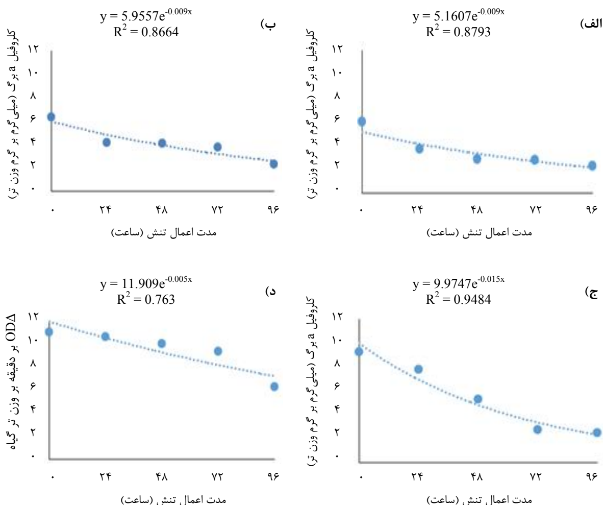
شکل ۶: تغییرات میزان کلروفیل a برگ (میلی گرم بر گرم وزن تر) کلزا طی دوره غرقابی (صفر، ۲۴، ۴۸، ۷۲ و ۹۶ ساعت) بر اساس مدل y = ae^{bx} در دماهای الف) ۱۰ درجه، ب) ۱۵ درجه، ج) ۲۰ درجه و د) ۲۵ درجه سانتی گراد
