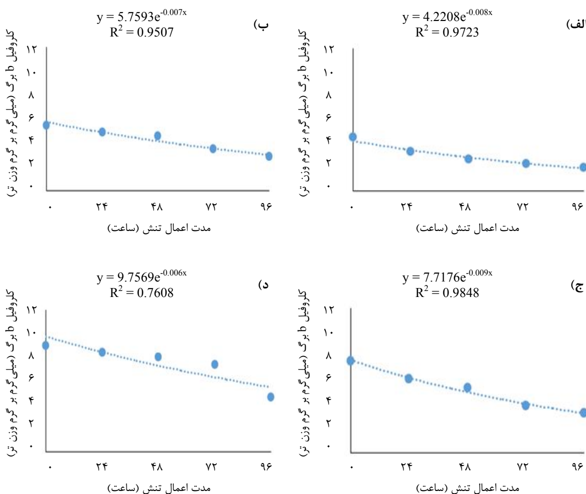
شکل ۷: تغییرات میزان کلروفیل b برگ (میلی‌گرم بر گرم وزن تر) کلزا طی دوره غرقابی (صفر، ۲۴، ۴۸، ۷۲ و ۹۶ ساعت) بر اساس مدل y = ae^{bx} در دماهای الف) ۱۰ درجه، ب) ۱۵ درجه، ج) ۲۰ درجه و د) ۲۵ درجه سانتی‌گراد
