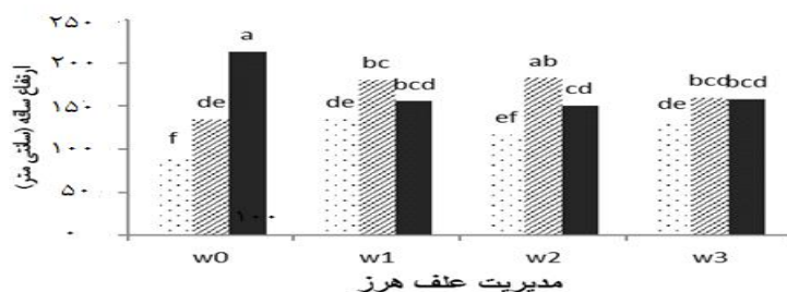
شکل ۱: اثر متقابل مدیریت علف هرز با نوع کوددهی بر ارتفاع ساقه گیاه نیشکر
