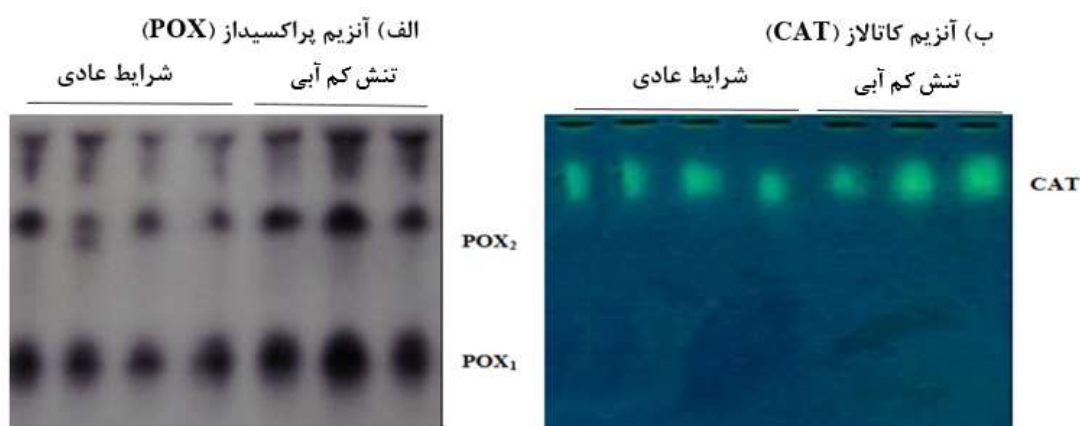
شکل ۲: فعالیت ایزوفرم‌های پراکسیداز و کاتالاز هیبریدهای ذرت تحت شرایط عادی و تنش کم آبی روی ژل پلی-آکریلامید
