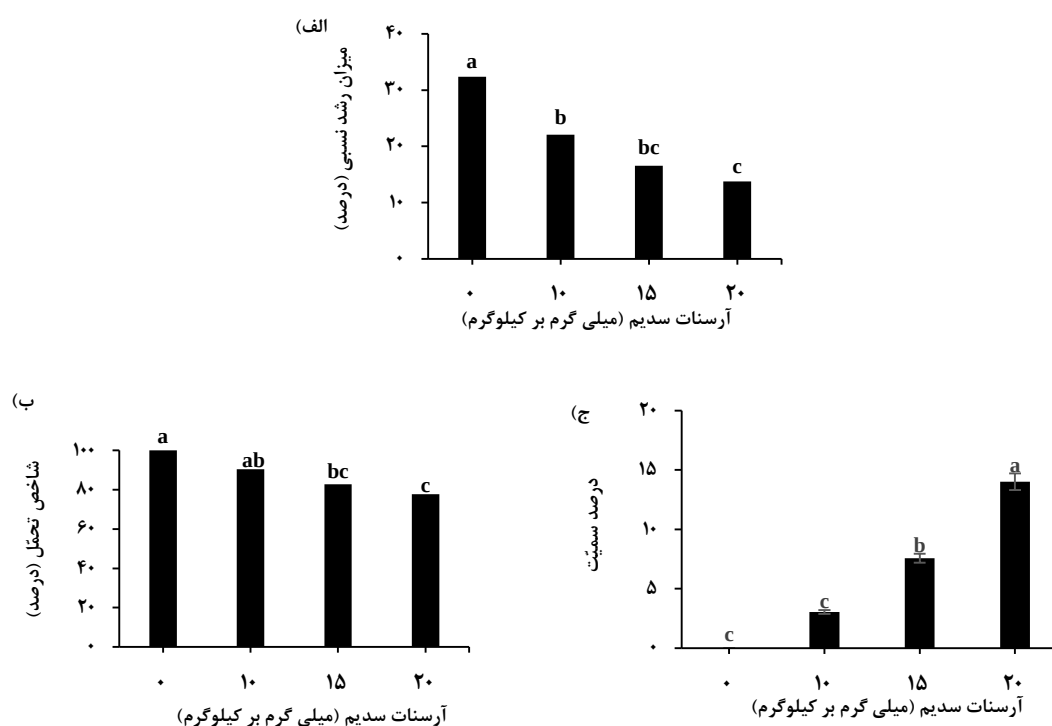
شکل ۱: نمودارهای مقایسه اثر غلظت‌های مختلف محلول آرسنات سدیم بر میزان رشد نسبی (الف)، شاخص تحمل (ب)
