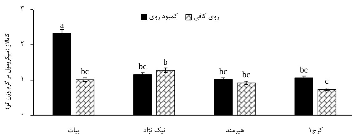
شکل ۳: مقایسه میانگین برهمکنش سطوح روی × رقم بر فعالیت آنزیم کاتالاز در گندم نان
