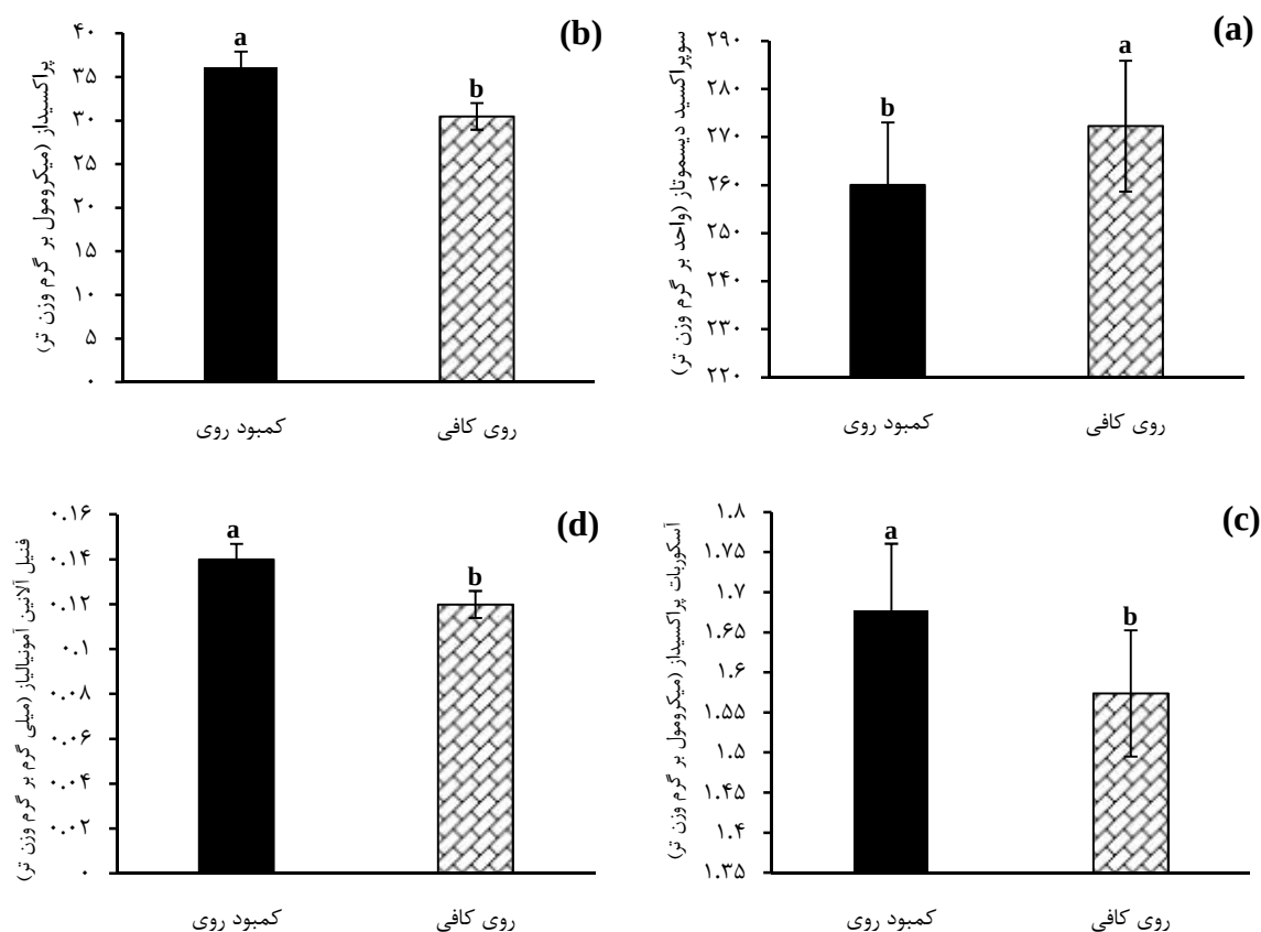
شکل ۱: مقایسه میانگین اثر اصلی سطوح روی بر فعالیت آنزیم‌های سوپراکسید دیسموتاز (a) پراکسیداز (b)، آسکوربات پراکسیداز (c) و فنیل آلانین آمونیالیز (d) در گندم نان
