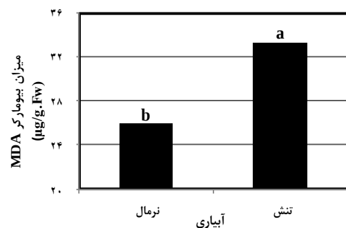
شکل ۳: اثر آبیاری بر بیومارکر MDA
