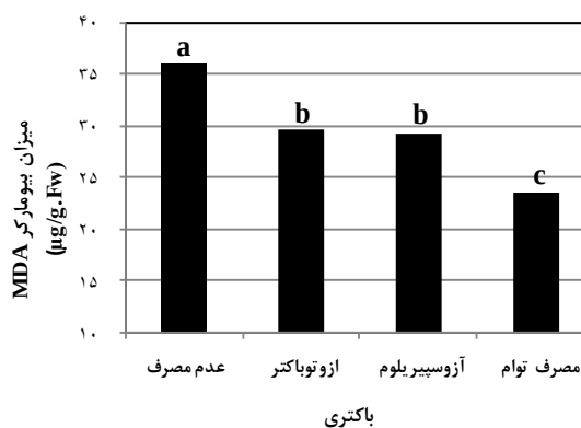
شکل ۶: اثر باکتری بر میزان بیومارکر MDA
