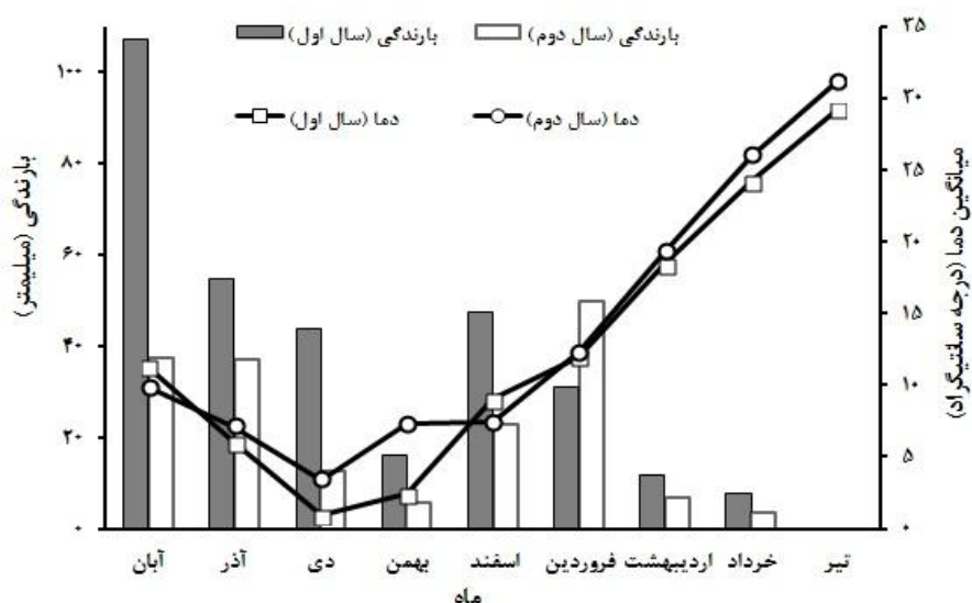
شکل ۱: میانگین بارندگی (میلی‌متر) و دمای (درجه سانتی‌گراد) ماهانه در طول فصول زراعی سال‌های آزمایش (۱۳۹۲-۹۳ و ۱۳۹۳-۹۴) (سازمان هواشناسی کشور)
