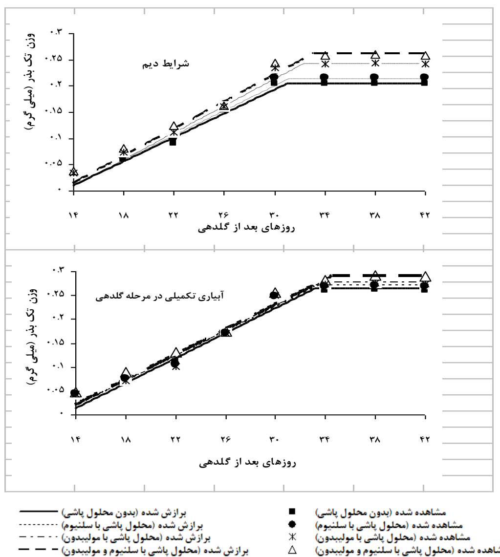
شکل ۱: تاثیر آبیاری تکمیلی و محلول‌پاشی سلیوم و مولیبدن بر روند پرشدن دانه عدس دیم
